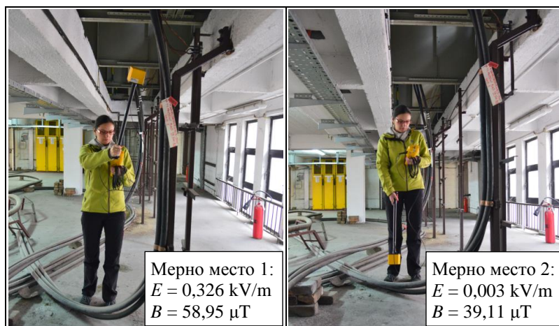
СЛИКА 11 – ПОЗИЦИЈЕ МЕРНИХ МЕСТА 1 И 2 И РЕЗУЛТАТИ МЕРЕЊА ( I = 100 \text{ A} )
