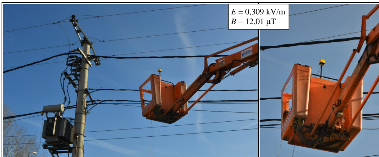
СЛИКА 8 – ПОЗИЦИЈА МЕРНОГ МЕСТА (ИСПОД 10 KV СКС-А) И РЕЗУЛТАТИ МЕРЕЊА ( H = 7 \text{ M} ; H_K = 5,3 \text{ M} ; H_S = 1,7 \text{ M} )
